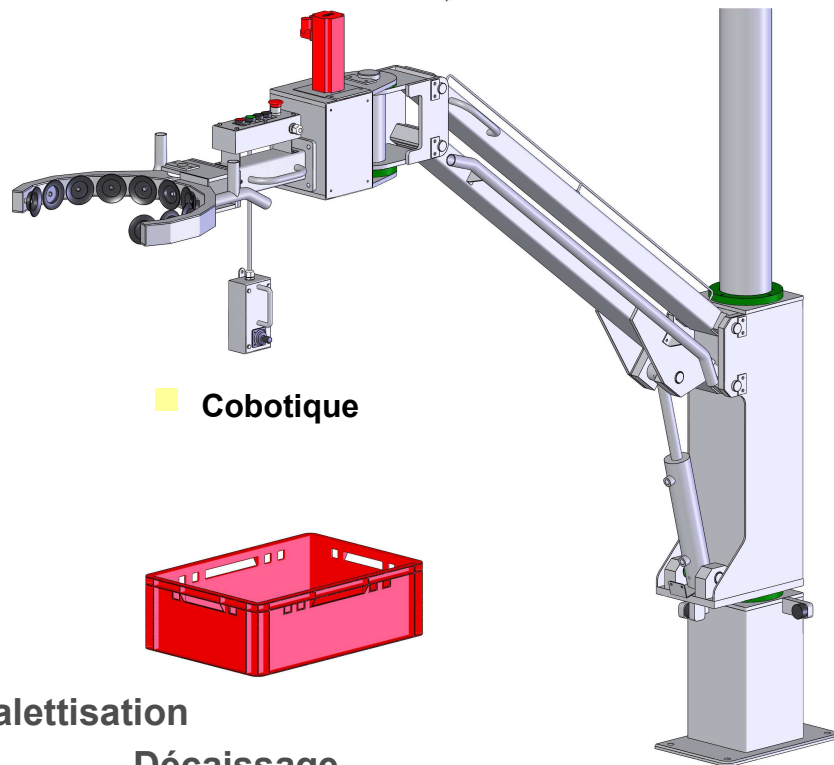
■ Bras de chargement
