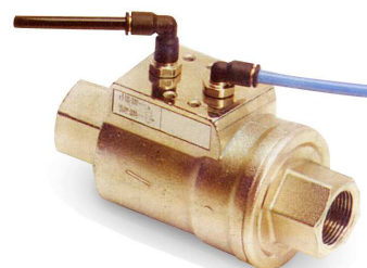
■ Vannes axiales pneumatiques Normalement ouvertes, normalement fermées ou double effet Ø 3/8 " à 2"
